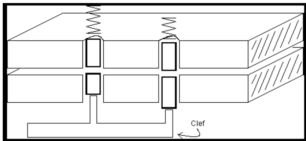
Schéma 3.2: (a) La clef lève les goupilles
